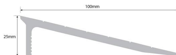
ST 100-25 Ramp
